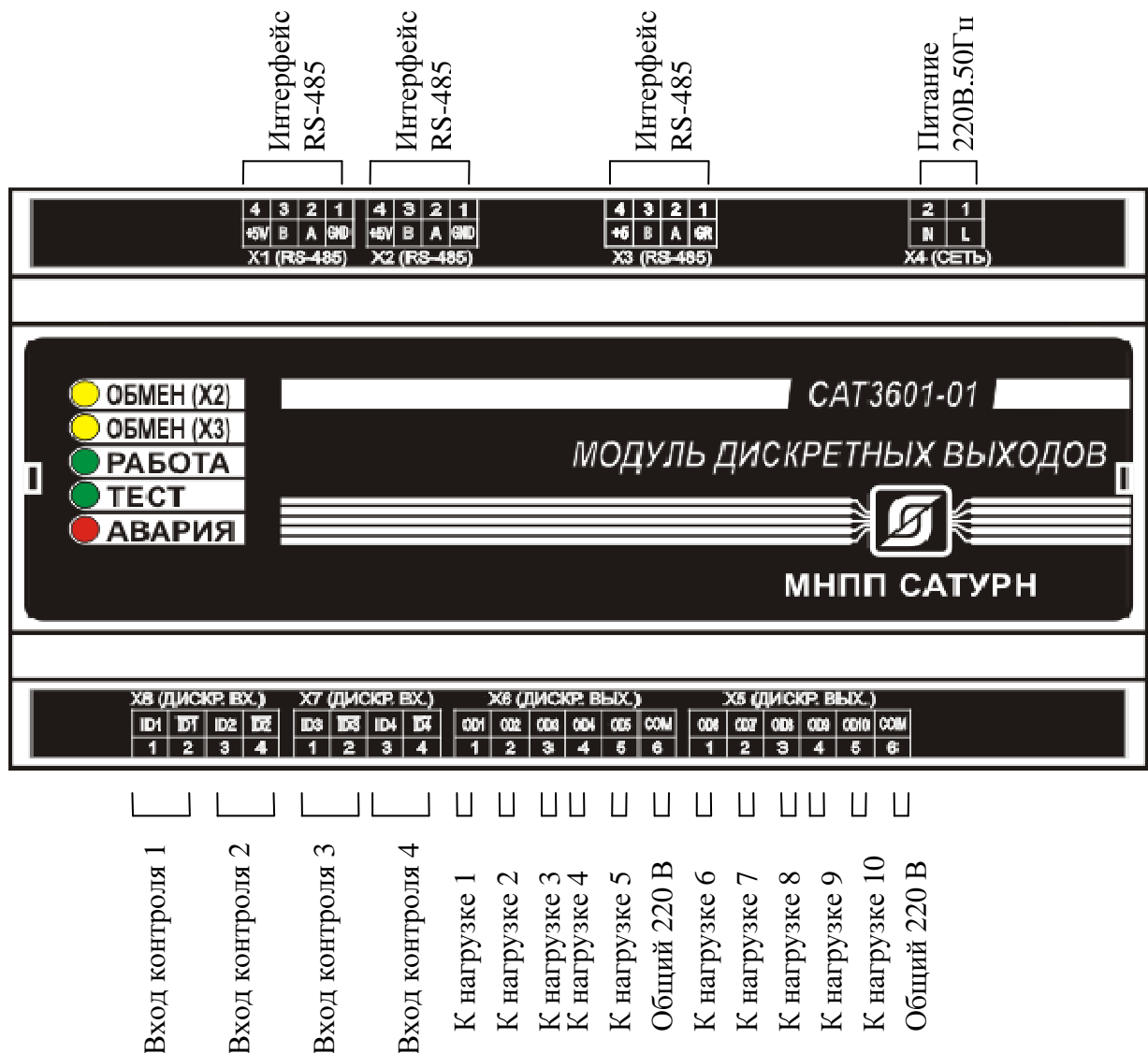
Рисунок 4 - Расположение разъёмов на плате САТ3601-01
