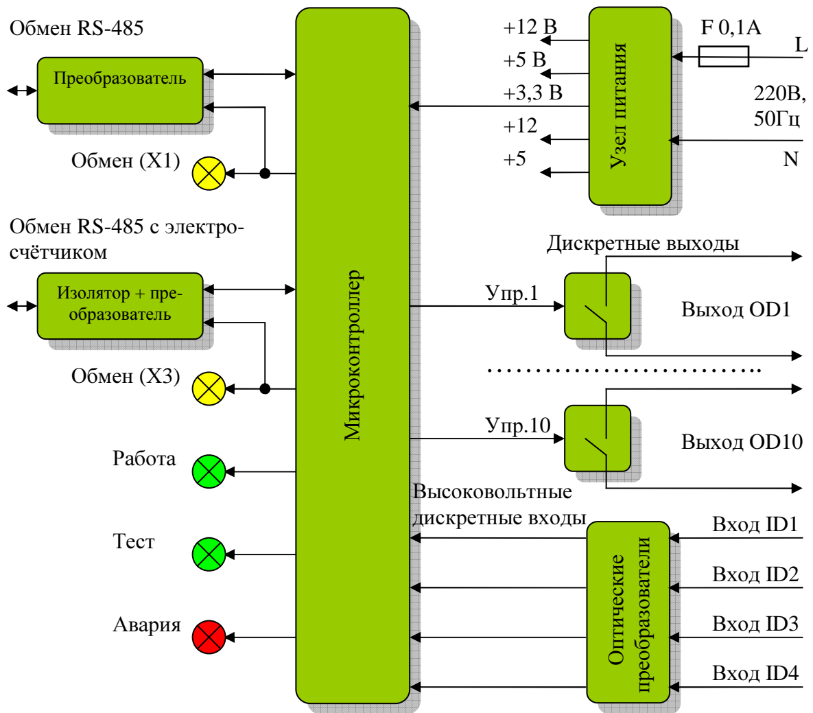
Рисунок 2 - Структурная схема САТ3601-01
