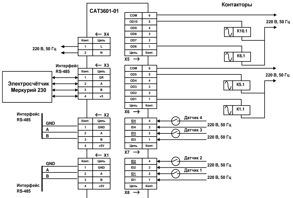
Рисунок 5 - Электрическая принципиальная схема подключения САТ3601-01 (типовая)
