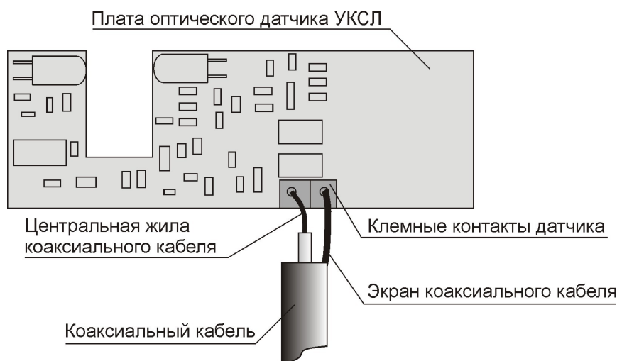
Рисунок 20 – Подсоединение датчика ДСЛ
