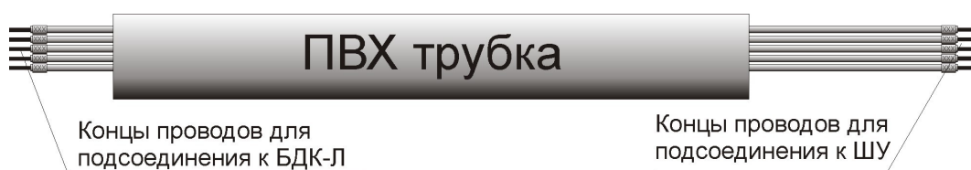
Рисунок 11 – Соединительный кабель «БДК-Л – ШУ лифта»
