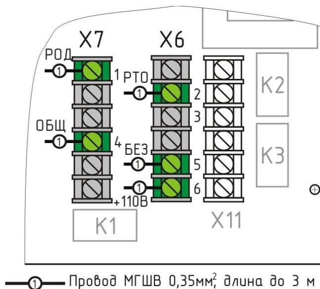
Рисунок 12 - Подключение цепей УБ
