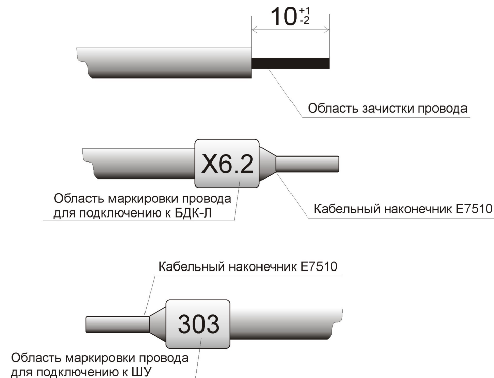
Рисунок 10 – Зачистка проводов, установка кабельного наконечника и маркировка проводов
