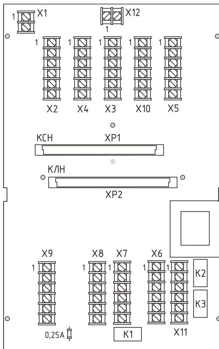
Рисунок 21- Расположение разъемов на коммутационной плате БДК-Л-4М2, БДК-Л-3М2
