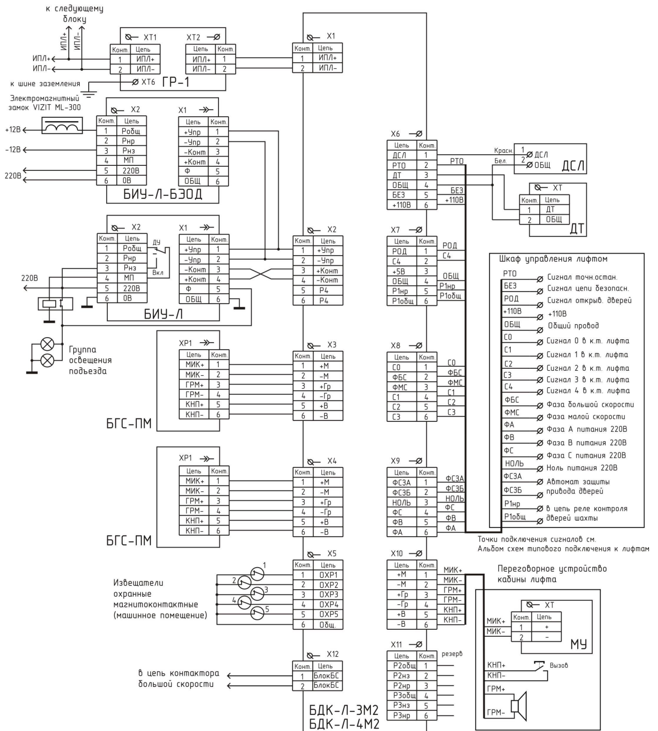
Рисунок 22 - Электрическая схема подключения БДК-Л-3М2, БДК-Л-4М2
