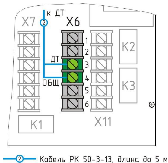
Рисунок 19 - Подключение датчика ДТ
