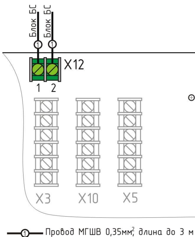
Рисунок 13 - Подключение цепи блокировки большой скорости
