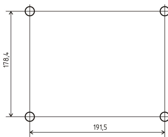
Рисунок 3 - Разметка для крепления блока БДК-Л-4М2, БДК-Л-3М2
