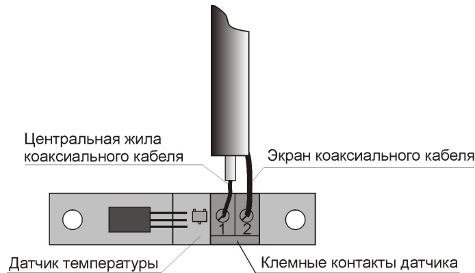
Рисунок 18 – Подсоединение датчика температуры
