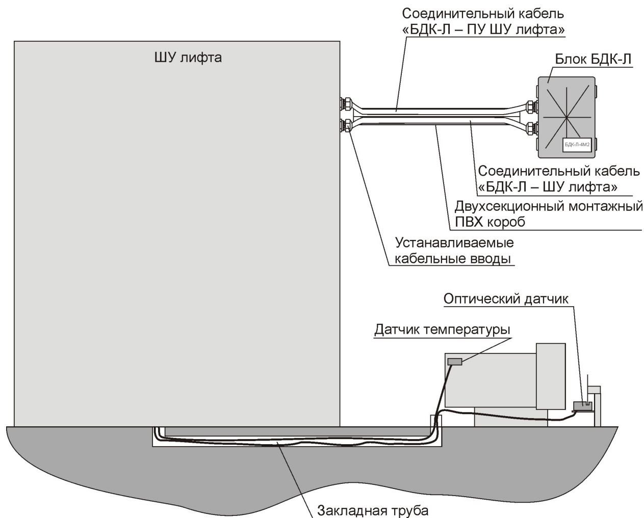
Рисунок 9 – Подсоединение БДК-Л-4М2, БДК-Л-3М2 к ШУ лифта
