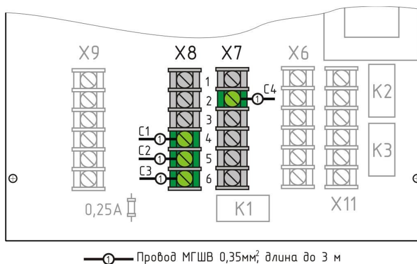
Рисунок 15 - Подключение цепей С0-С4
