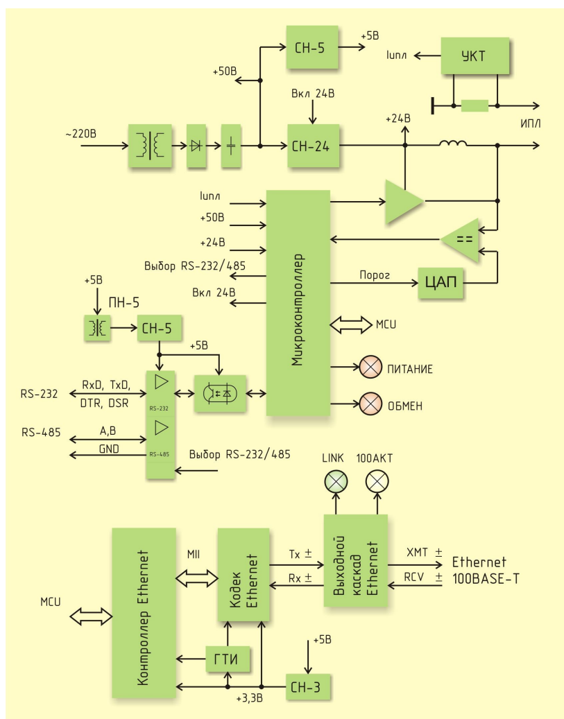
Рисунок 3 - Функциональная схема БКД-МЕ
