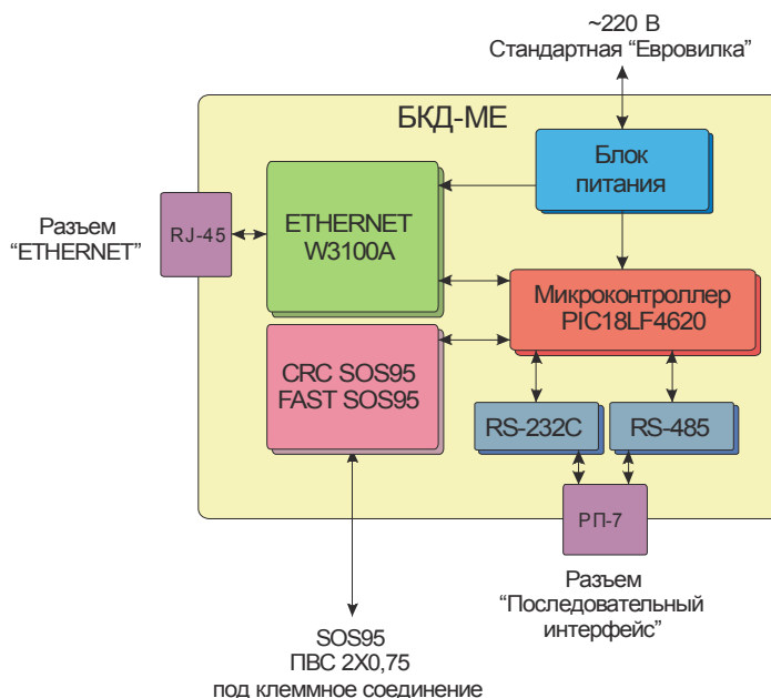
Рисунок 2 - Структурная схема БКД-МЕ
