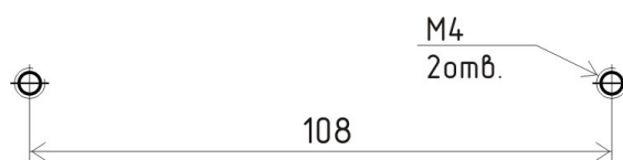
Рисунок 5 - Шаблон для сверления отверстий крепления
