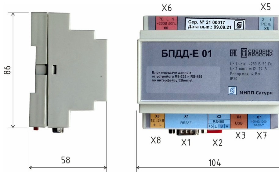
Рисунок 2 - Габаритные размеры БПД-Е 01
