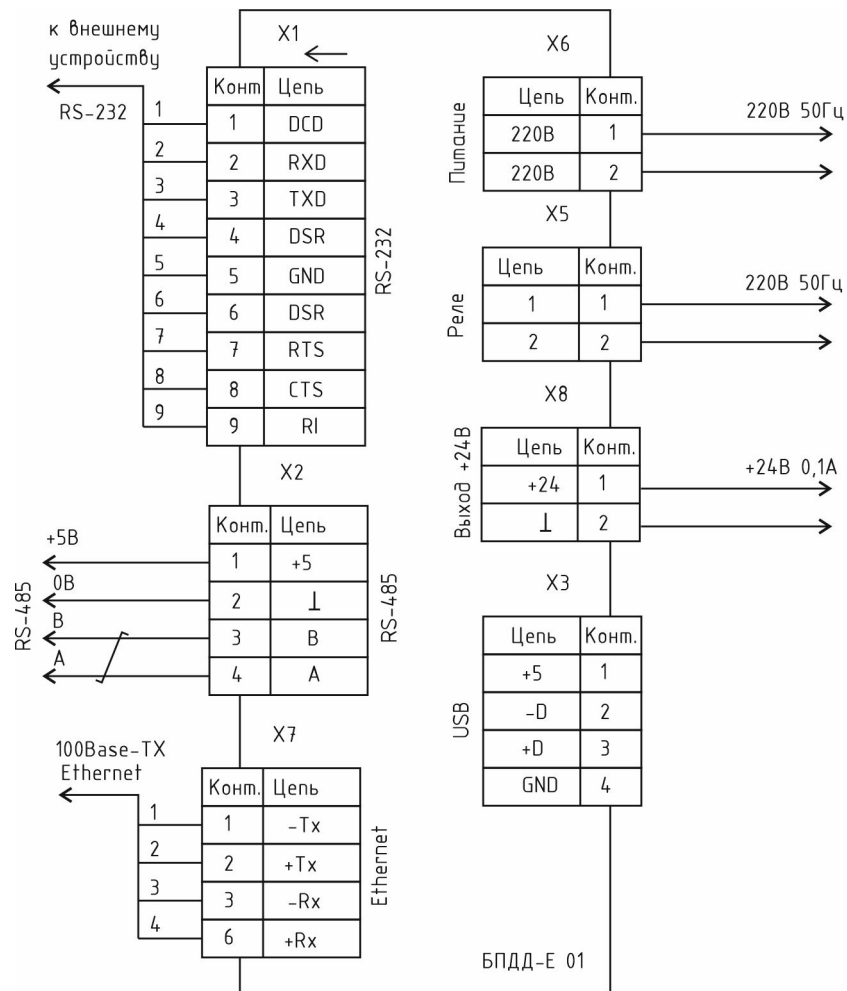
Рисунок 4 - Электрическая схема подключения внешних цепей БПДД-Е 01
