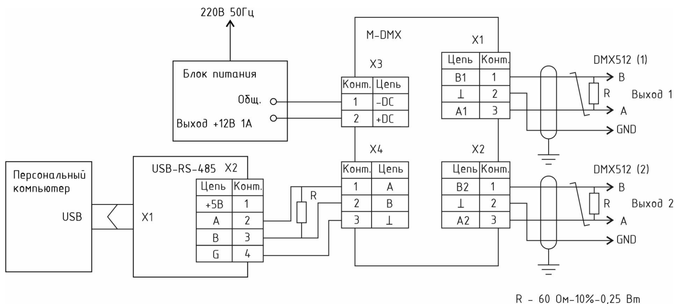
Рисунок 5 – Подключение модуля к персональному компьютеру
