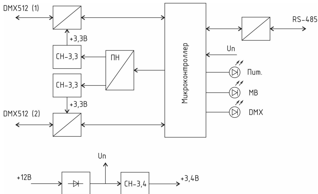
Рисунок 4 – Функциональная схема модуля
