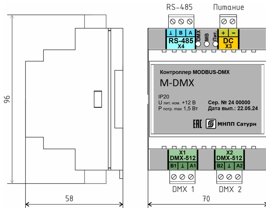
Рисунок 2 - Габаритные размеры модуля
