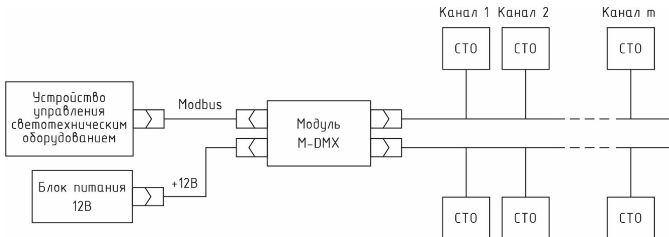
Рисунок 1 – Структурная схема управления светотехническим оборудованием
