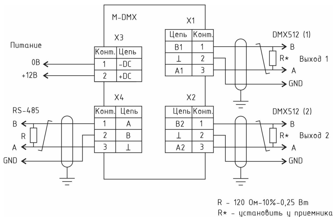
Рисунок 3 – Схема подключения модуля
