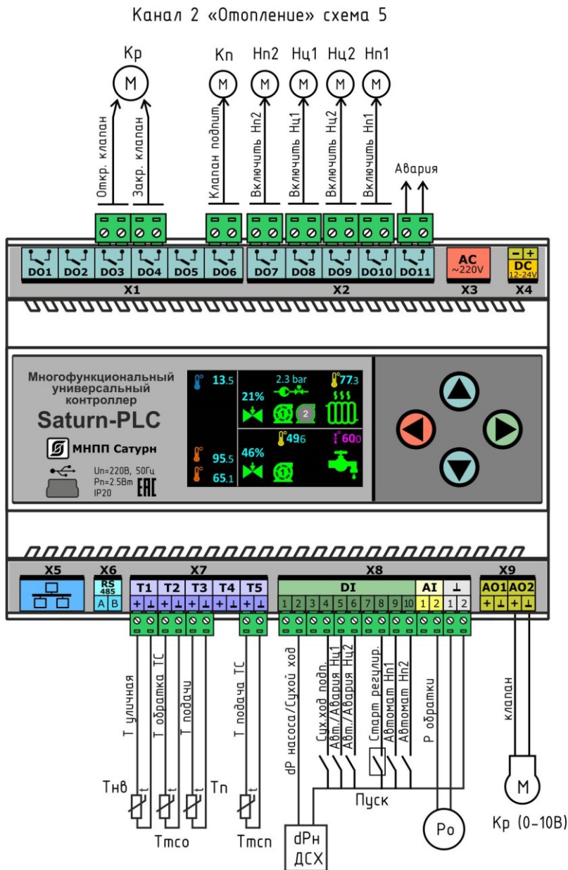
Рисунок 11 - Схема подключения датчиков и исполнительных механизмов в режиме «Отопление» (схема 5) для канала регулирования №2
