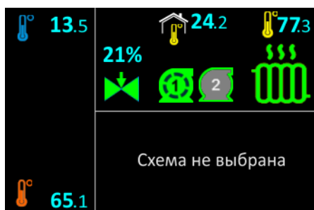
Рисунок 30 - Пример индикации режима «Независимое отопление (3)»
