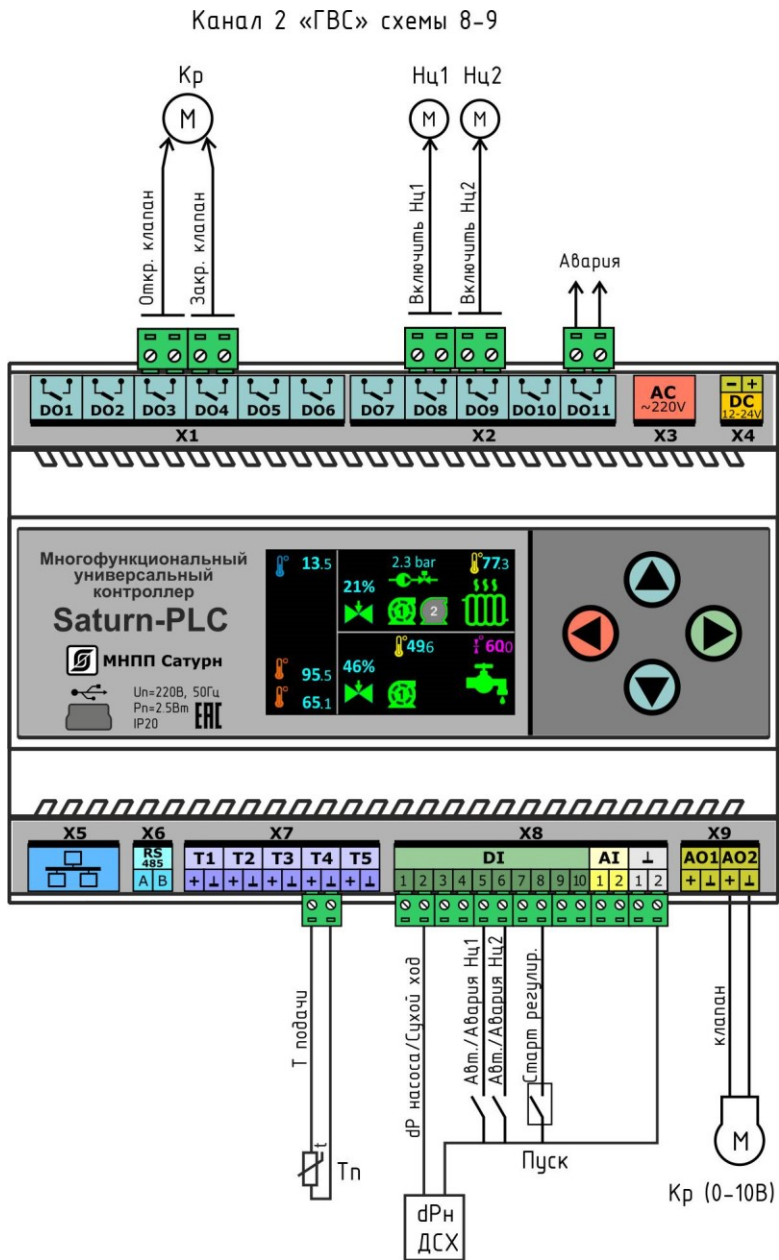
Рисунок 17 - Функциональная схема контроллера в режиме «ГВС (схемы 8, 9)», канал регулирования №2
