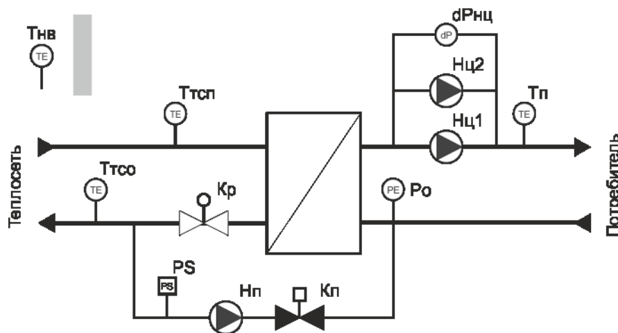
Рисунок 25 - Мнемосхема «Независимое отопление (1)»
