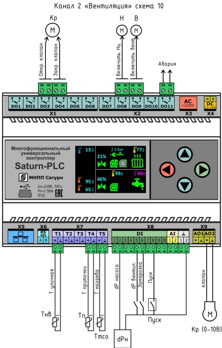
Рисунок 22 - Структурная схема системы регулирования в режиме «Вентиляция», канал регулирования №2
