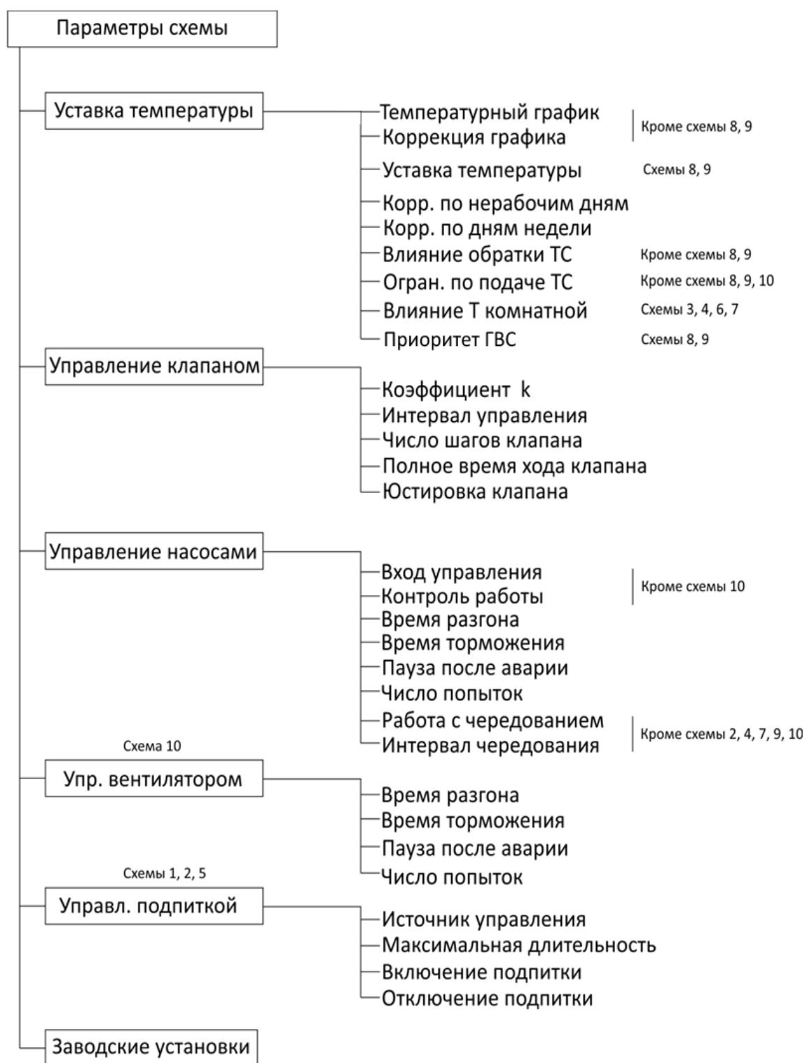
Рисунок 23 - Блок-схема пунктов меню «Параметры»
