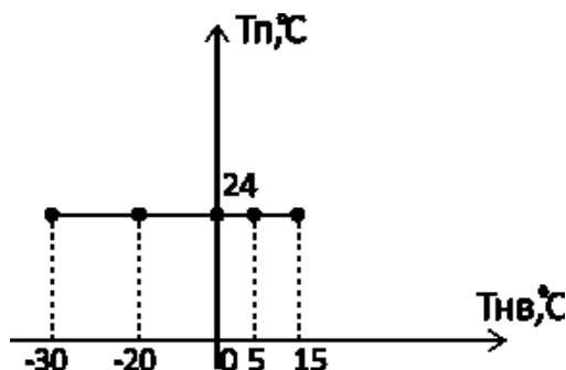
Рисунок 19 - Температурный график T_p=f(T_{нв})
