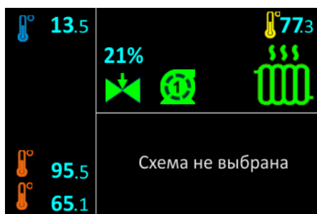
Рисунок 33 - Пример индикации режима - «Независимое отопление (4)»
