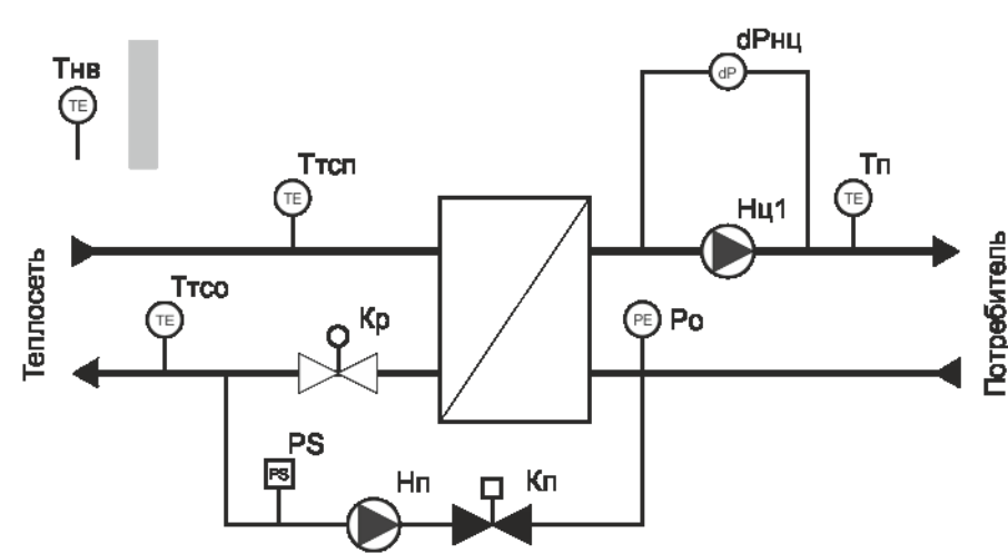
Рисунок 27 - Мнемосхема «Независимое отопление (2)»
