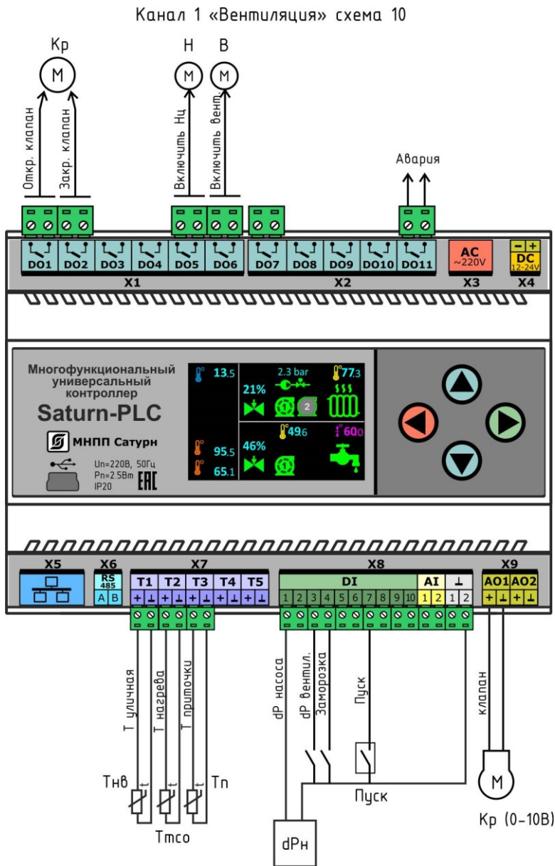
Рисунок 21 - Структурная схема системы регулирования в режиме «Вентиляция», канал регулирования №1
