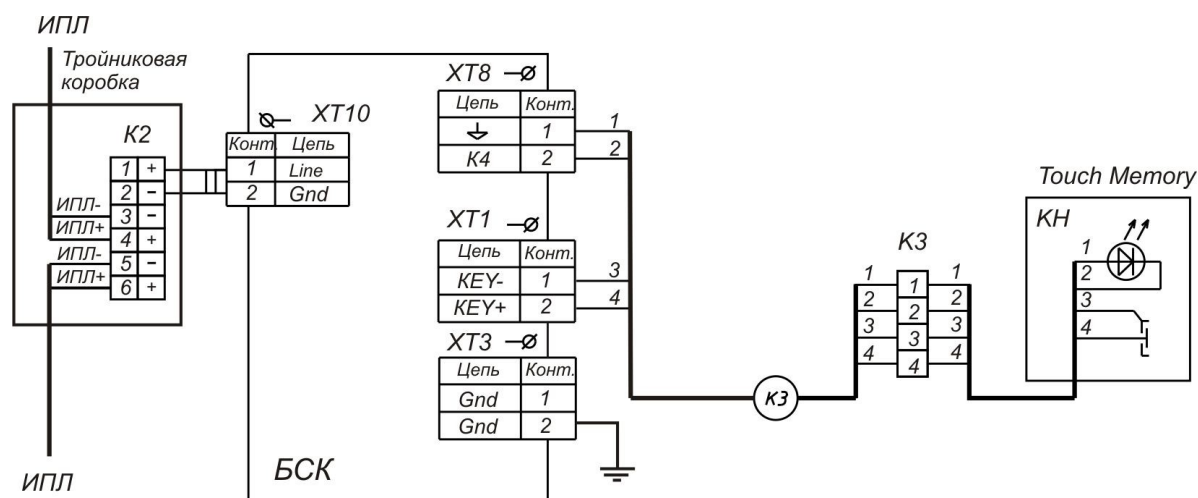
Рисунок 3 - Электрическая схема подключения считывателя к БСК
