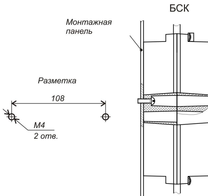
Рисунок 4 - Крепление БСК в шкафу ОПС
