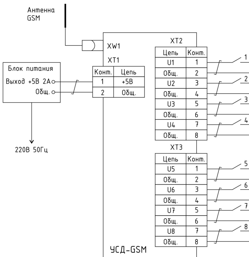
Рисунок 31 - Схема подключения датчиков с выходами «сухой контакт» и внешнего блока питания
