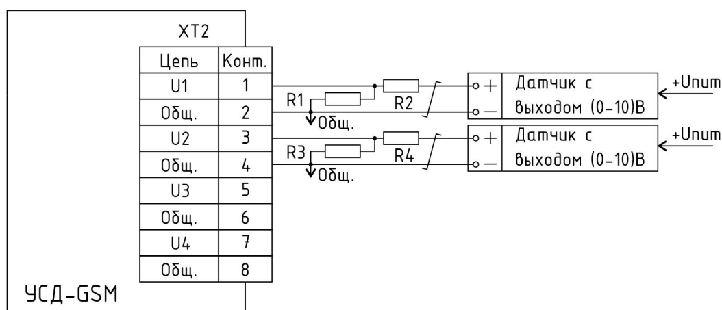
Рисунок 32 - Схема подключения датчиков с аналоговым выходом (0-10) В с питанием от сети
