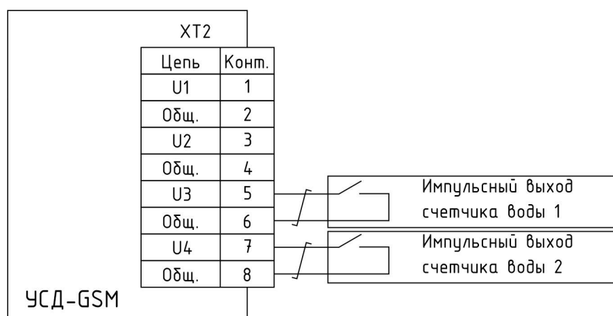
Рисунок 36 - Схема подключения датчиков с выходами «сухой контакт» и внешнего блока питания
