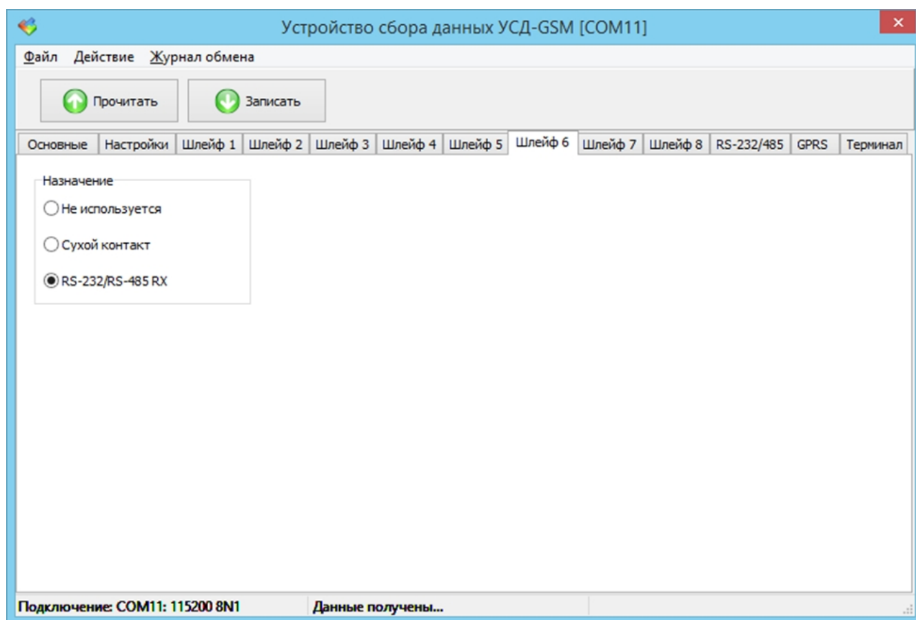
Рисунок 17 – Вкладка настройки шлейфа 6 окна конфигурации УСД-GSM
