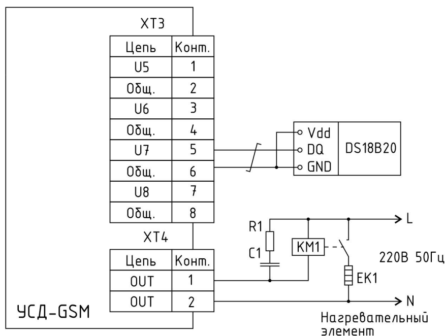
Рисунок 37 - Схема подключения преобразователя температуры DS18S20 (DS18B20) в режиме термостата
