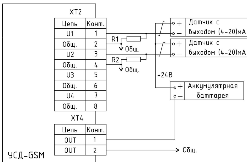
Рисунок 35 - Схема подключения датчиков с аналоговым выходом (4-20) мА для автономного электропитания
