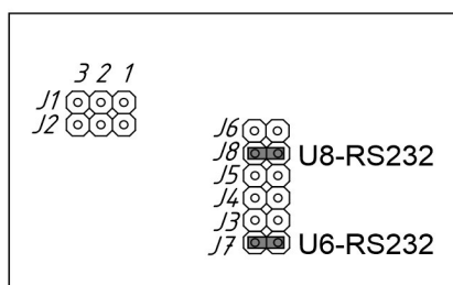
Рисунок 44 – Установка перемычек J7, J8 для включения интерфейса RS-232
