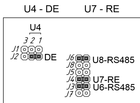
Рисунок 40 – Установка перемычек J1-J8 для сигналов U4, U7 для интерфейса RS-485
