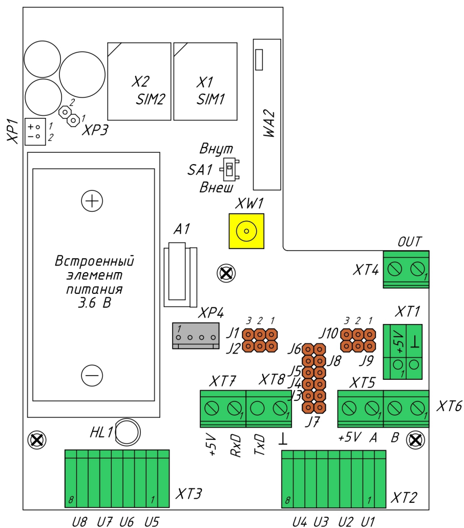
Рисунок 4 – Расположение разъемов устройства
