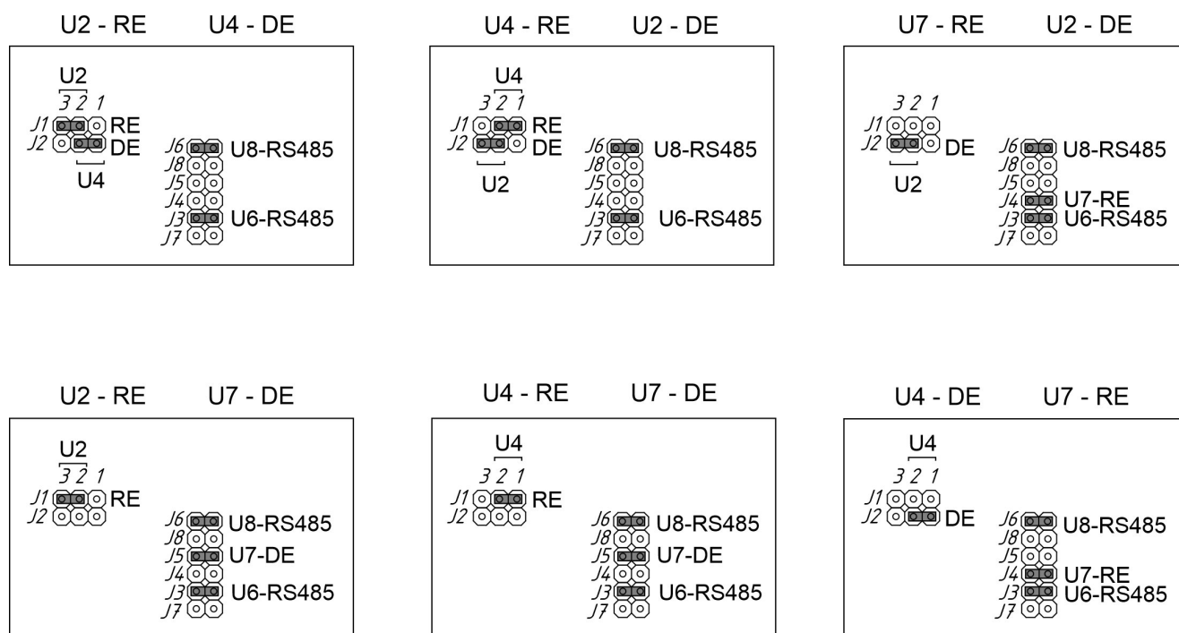
Рисунок 41– Примеры установки перемычек J1-J8 в зависимости от используемых сигналов U2, U4, U7 для интерфейса RS-485
