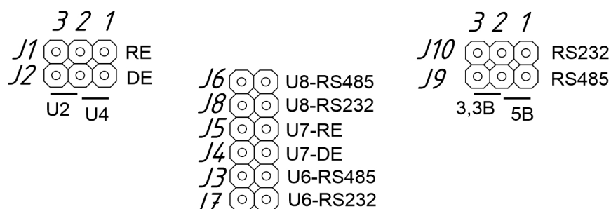
Рисунок 38 – Расположение перемычек J1–J10 на электронной плате
