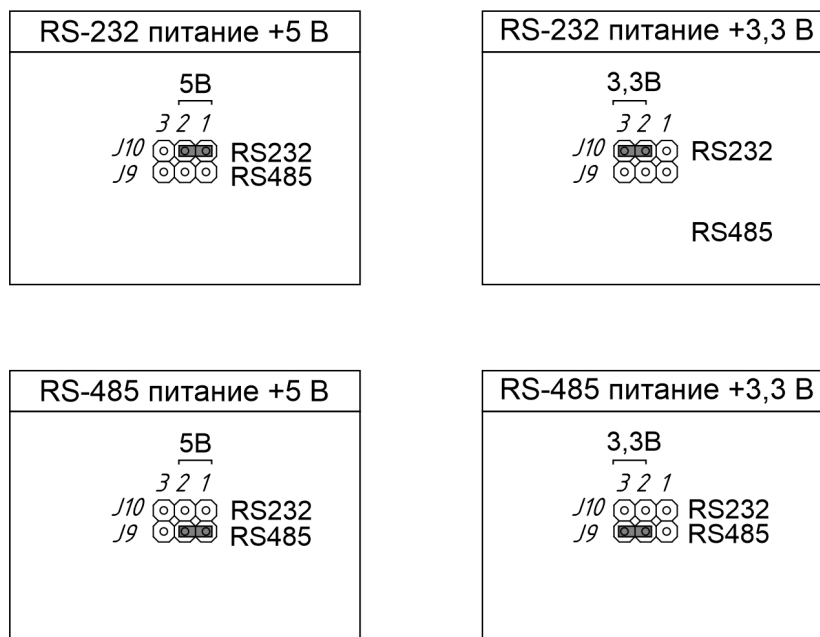
Рисунок 45 - Установка перемычек J9-J10 для выбора напряжения питания интерфейсов RS-485, RS-232
