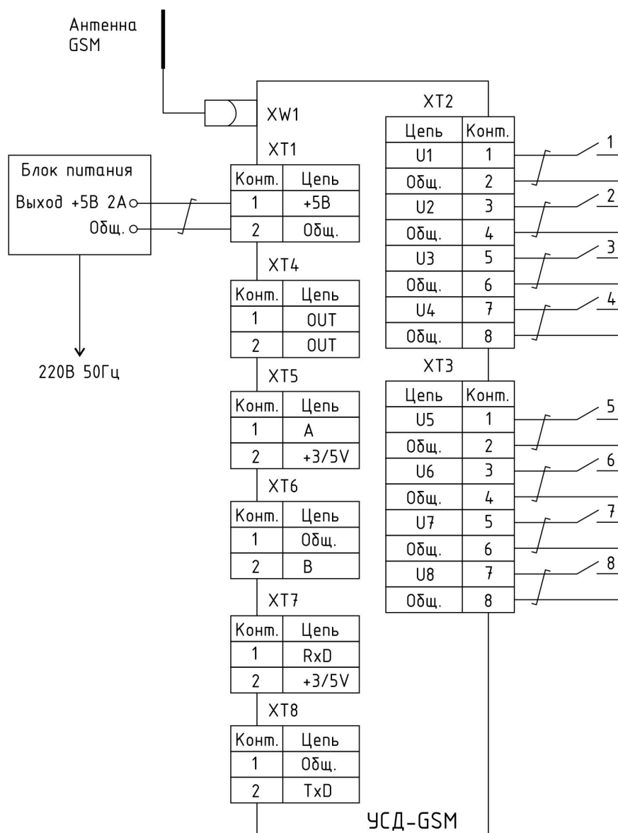
Рисунок 5 - Схема электрическая типового подключения устройства УСД-GSM
