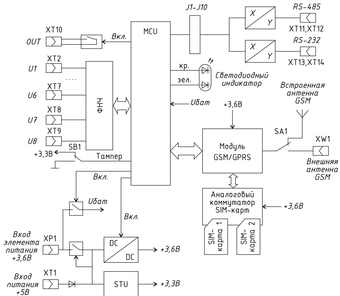
Рисунок 5 – Функциональная схема устройства УСД-GSM
