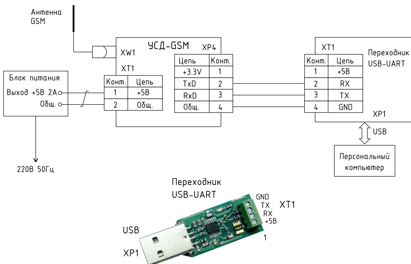
Рисунок 6 - Подключение УСД-GSM к переходнику USB-UART
