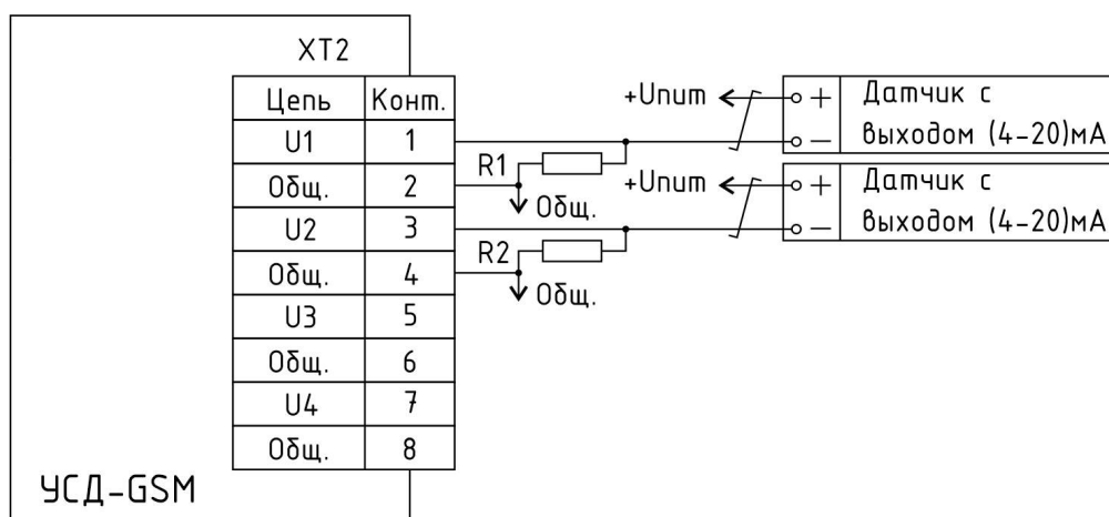
Рисунок 33 - Схема подключения датчиков с аналоговым выходом (4-20) мА
