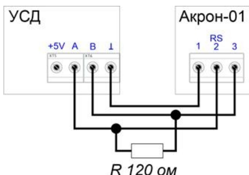
Рисунок 27 – Подключение УСД-GSM к прибору «Акрон-01»
