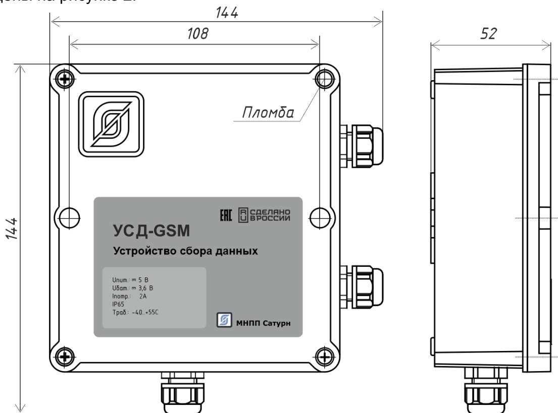
Рисунок 2 - Габаритные размеры устройства сбора данных УСД-GSM
