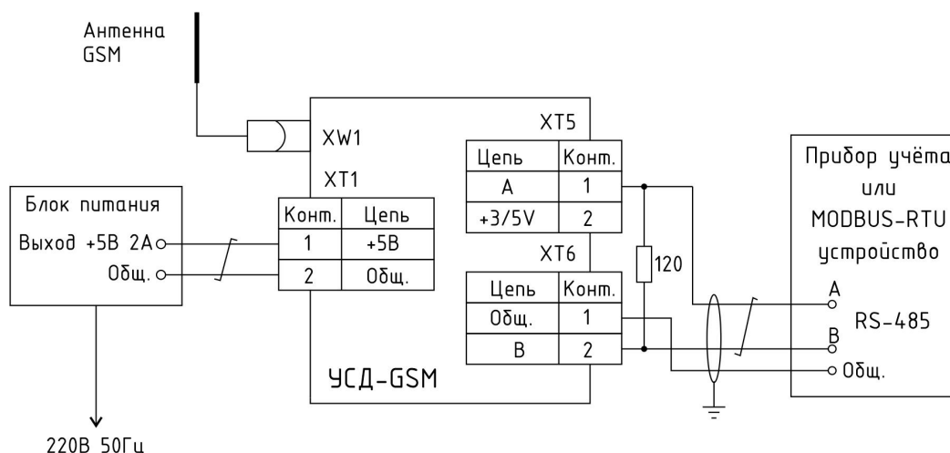
Рисунок 39 - Схема подключения внешнего устройства по интерфейсу RS-485
