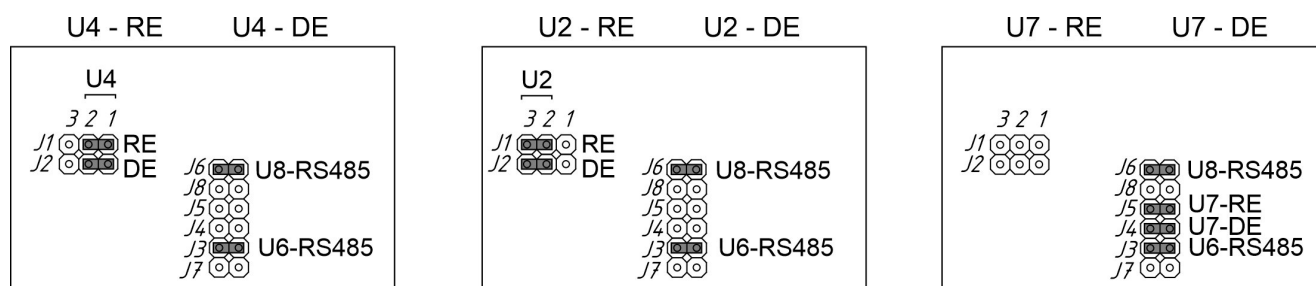
Рисунок 42 – Примеры установки перемычек J1-J8 в зависимости от используемых сигналов U2, U4, U7 для неотключаемого интерфейса RS-485
