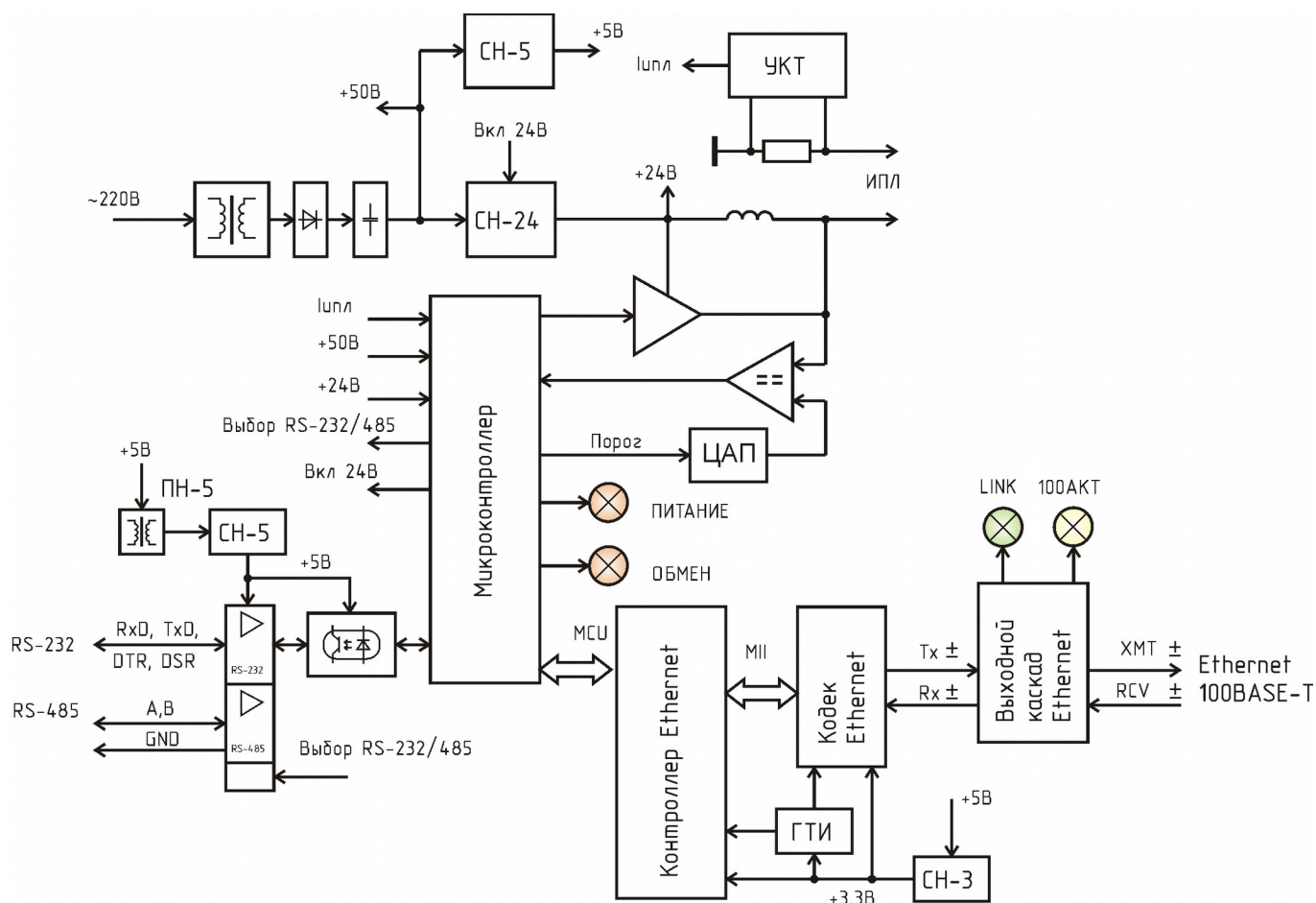
Рисунок 3 - Функциональная схема БКД-МЕ
