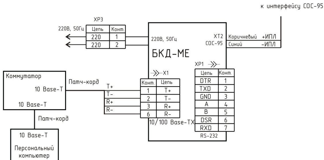
Рисунок 9 - Схема подключения БКД-МЕ к ПЭВМ по Ethernet
