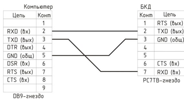
Соединительный кабель "Соединитель БКД - ЭВМ"
