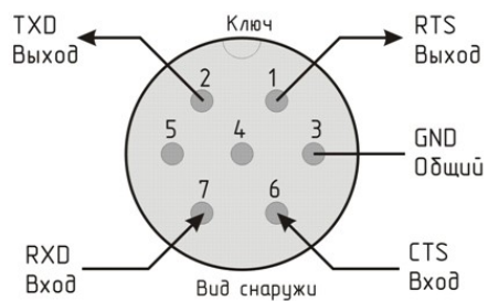
Разъем PC7TB-вилка на корпусе БКД-МЕ
