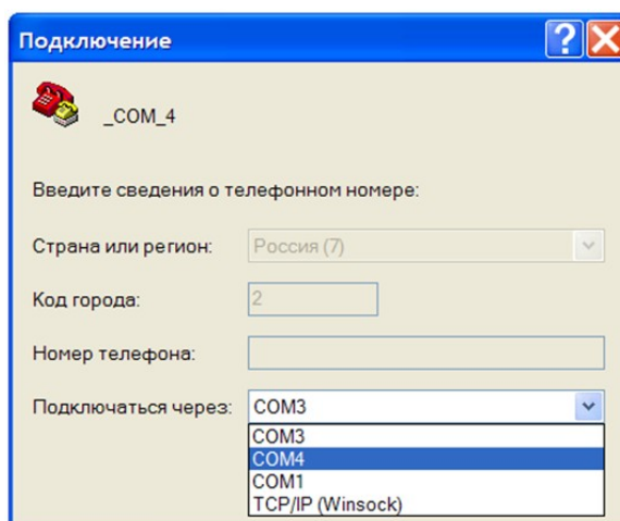
Рисунок 30 - Выбор порта
