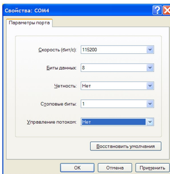
Рисунок 31 - Параметры порта
