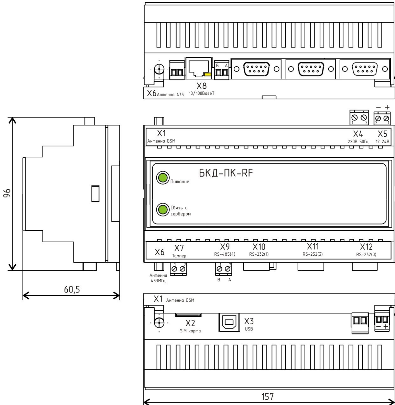
Рисунок 2 - Габаритные размеры БКД-ПК-RF
