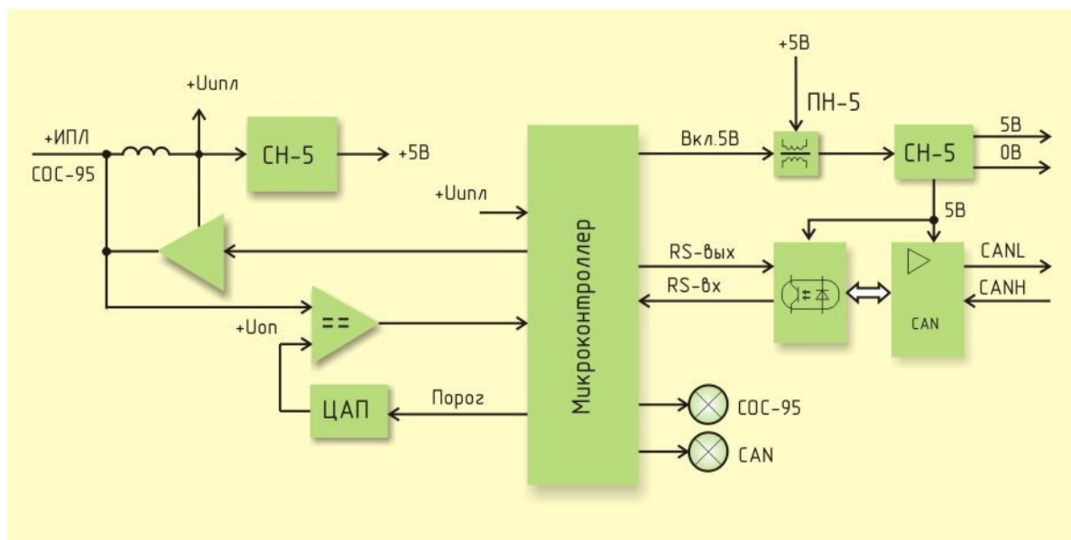
Рисунок 2 - Структурная схема БПДД-CAN
