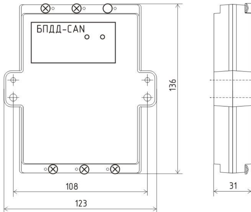
Рисунок 3 - Габаритные размеры БПДД-CAN
