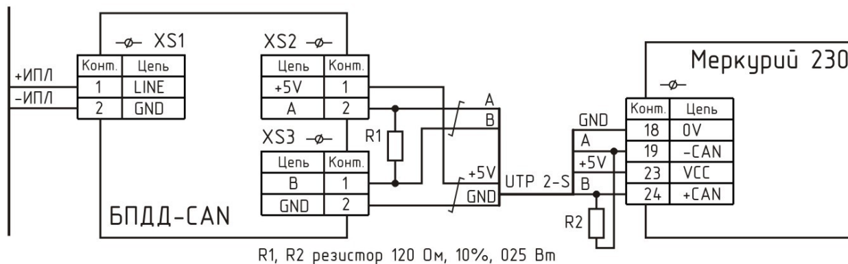
Рисунок 8 - Схема подключения электросчетчика Меркурий 230
