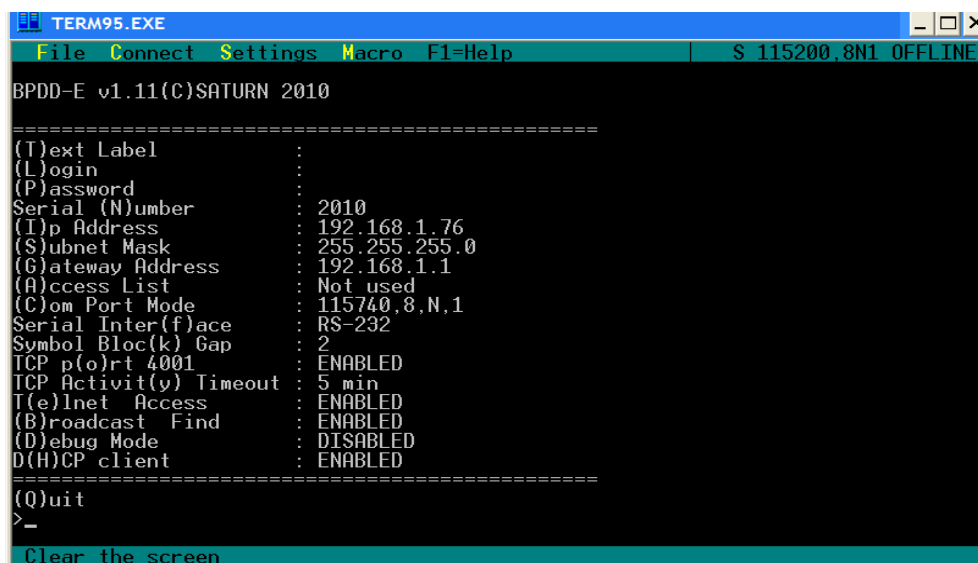
Рисунок 14 – Внешний вид окна терминала в режиме конфигурации по последовательному порту
