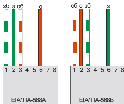
Рисунок 10 - Схемы заделки четырехжильного кабеля «витая пара»:
