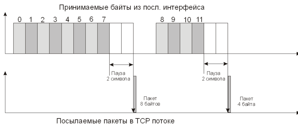
Рисунок 25 - Межблочный интервал 2 символа
