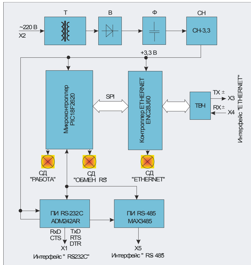
Рисунок 3 - Функциональная схема БПДД-Е
