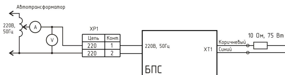
Рисунок 6 - Подключение приборов при проверке БПС
