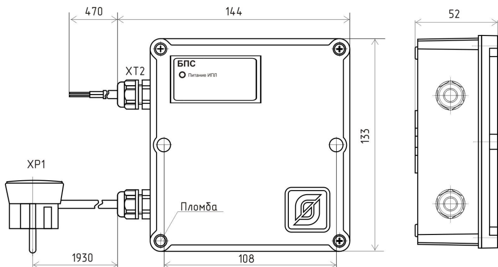
Рисунок 3 - Габаритные размеры БПС
