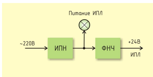
Рисунок 2 - Функциональная схема БПС
