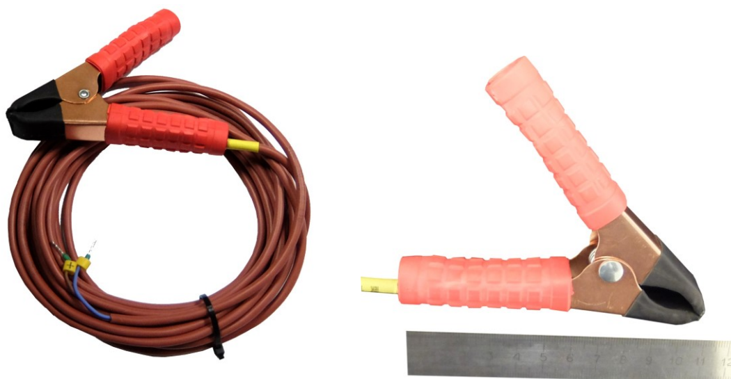
Рисунок 1 – Внешний вид датчика ТД-5
