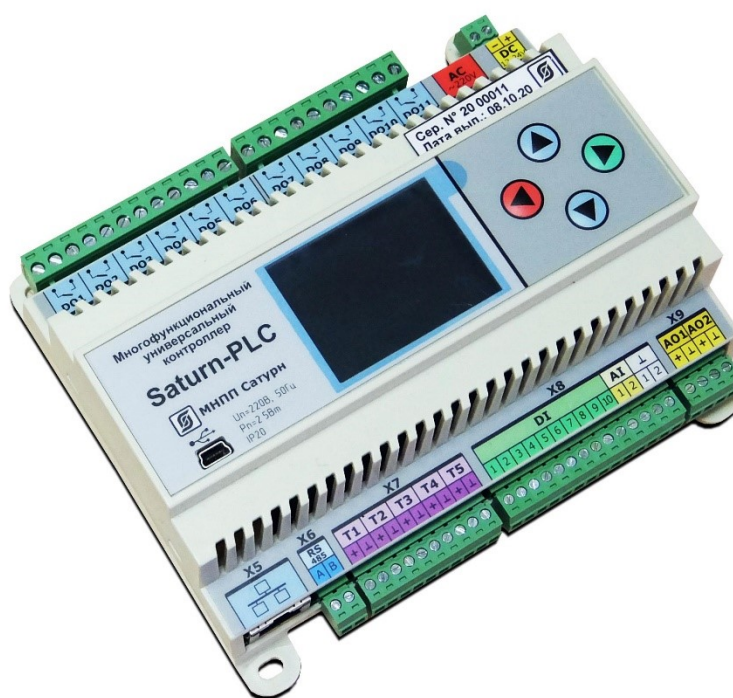
Рисунок 1 - Внешний вид контроллера «Saturn-PLC»
