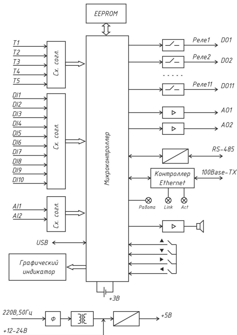
Рисунок 4 – Структурная схема контроллера «Saturn-PLC»
