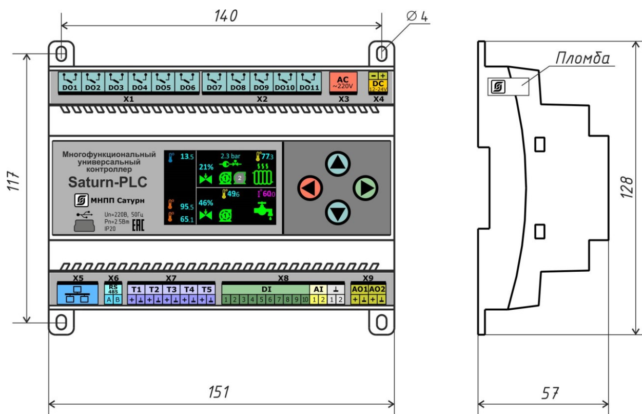
Рисунок 2 – Габаритные размеры контроллера «Saturn-PLC»
