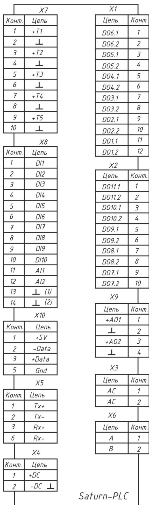
Рисунок 3 – Разъемы контроллера «Saturn-PLC»
